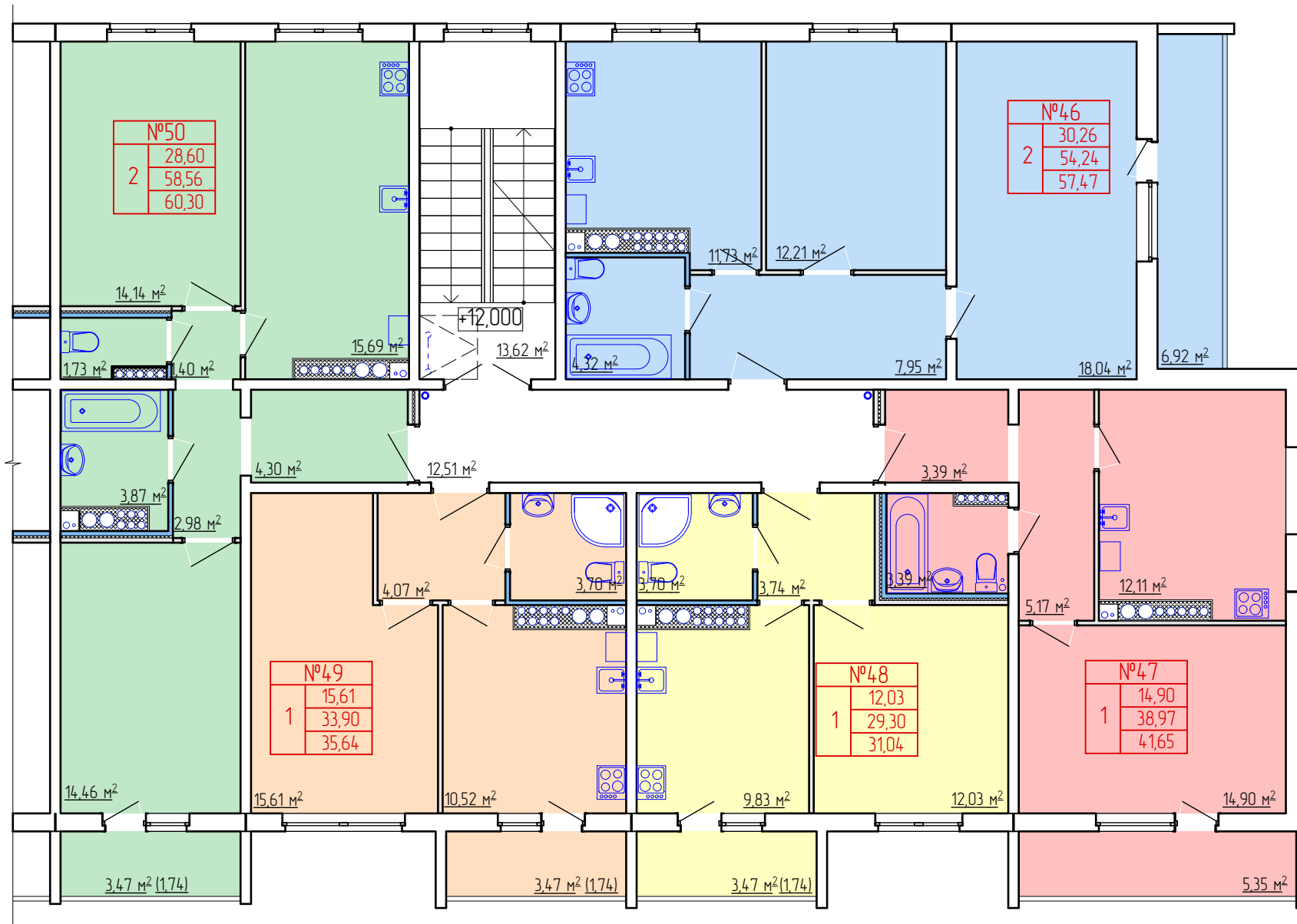
План пятого этажа. М 1:100
