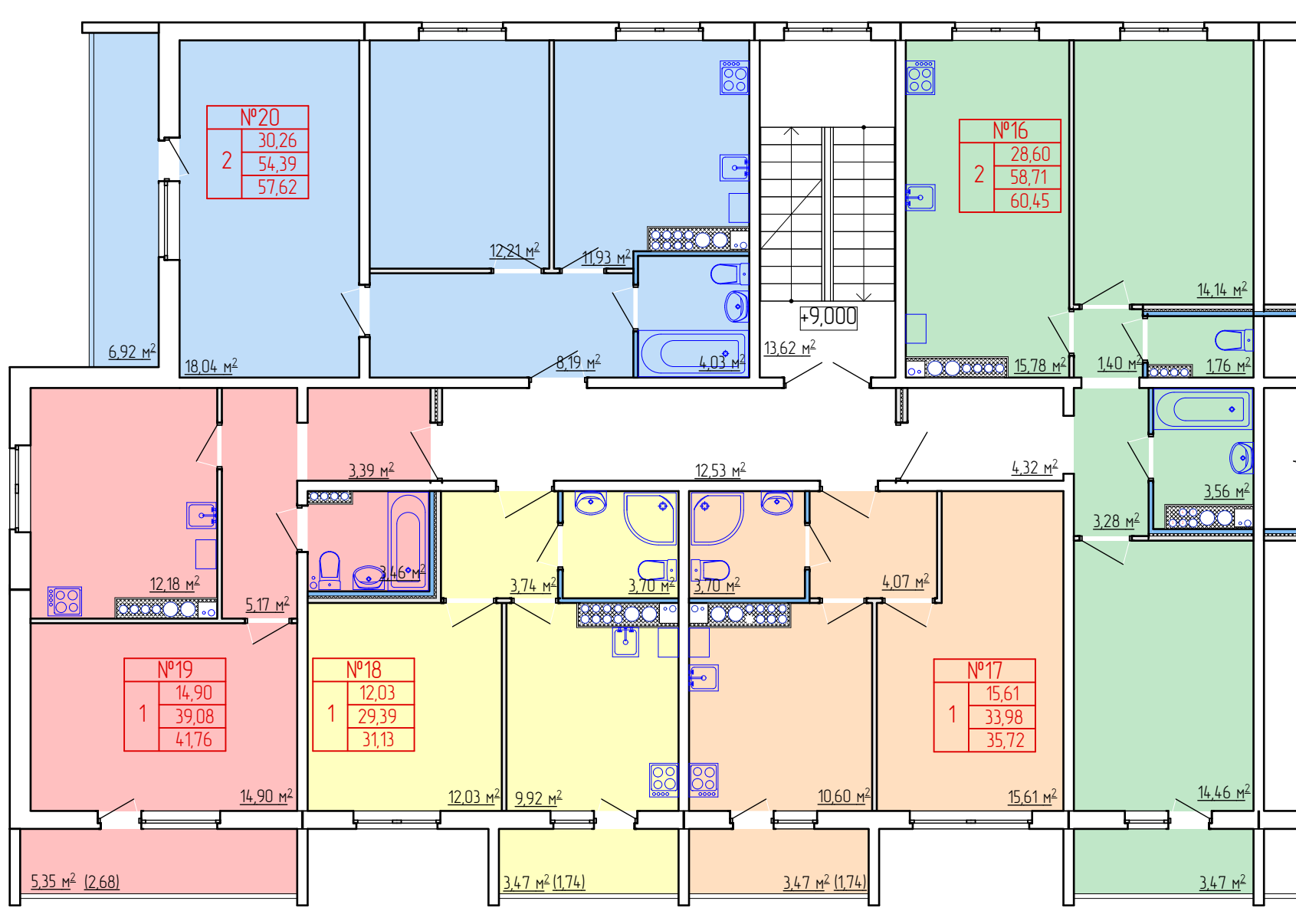
План четвертого этажа. М 1:100
