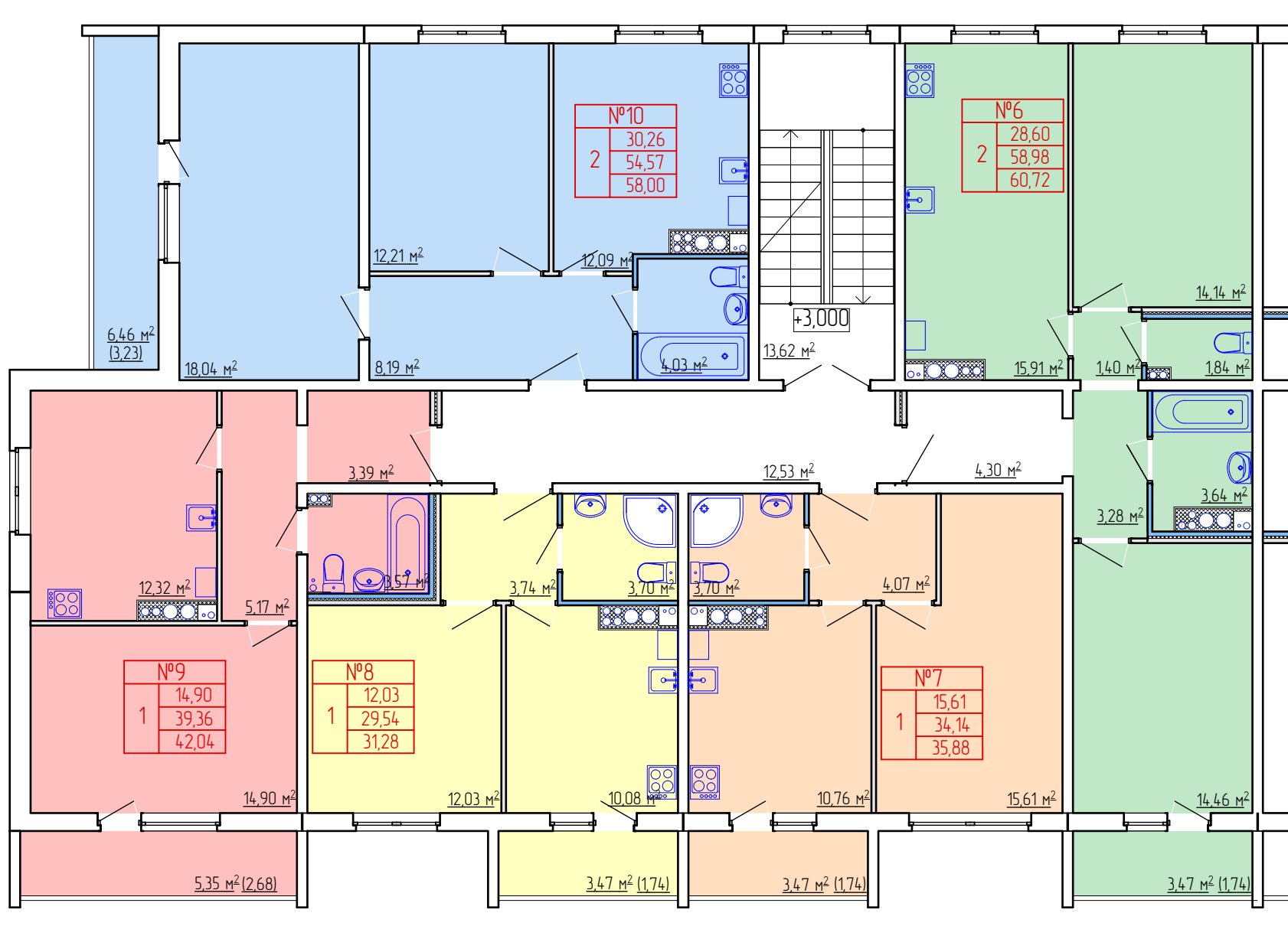
План второго этажа. М 1:100
